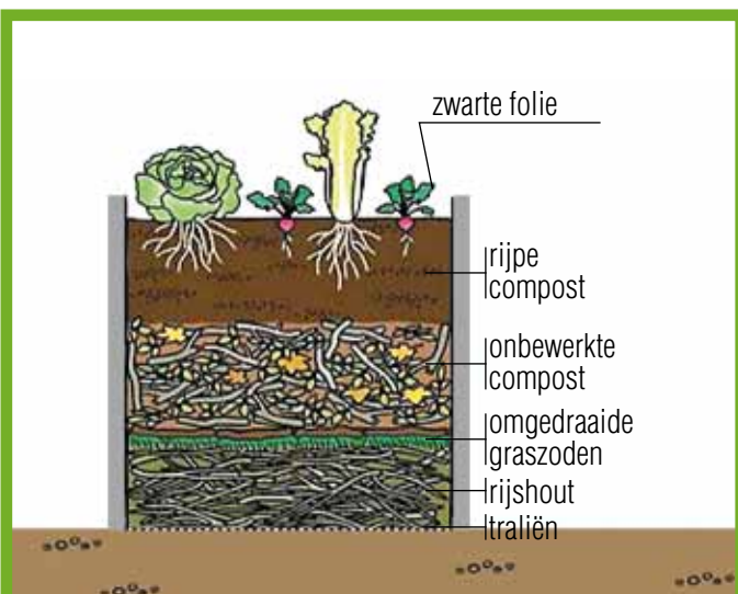
Dwarsdoorsnede van het verhoogde plantenbed.
